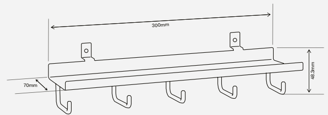
Dimensions
